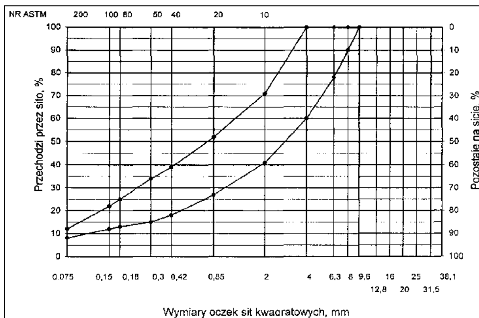
Rys. 3. Krzywe graniczne uziarnienia mieszanki mineralnej BA od 0 do 8mm, od 0 do 6,3 mm do warstwy ścieralnej nawierzchni drogi o obciążeniu ruchem nawierzchni drogi o obciążeniu ruchem KR1 lub
